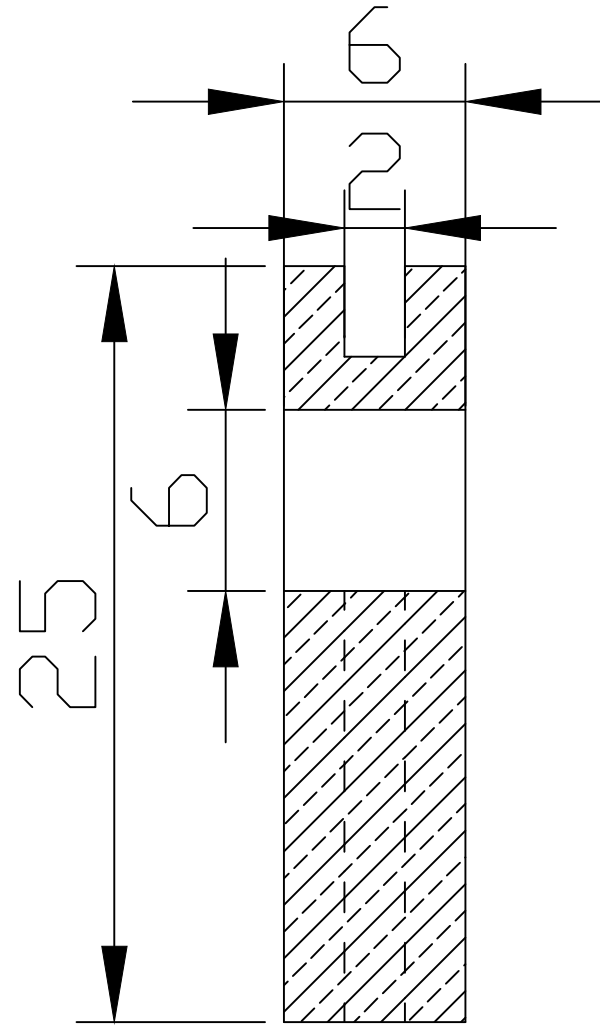
Sezione A-A
